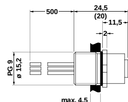
Montagekontakt M 12 x 1, med låsmutter (klamtermått: montagekontakt utan låsmutter), hona
