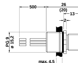
Montagekontakt M 12 x 1, med låsmutter (klamtermått: montagekontakt utan låsmutter), hane
